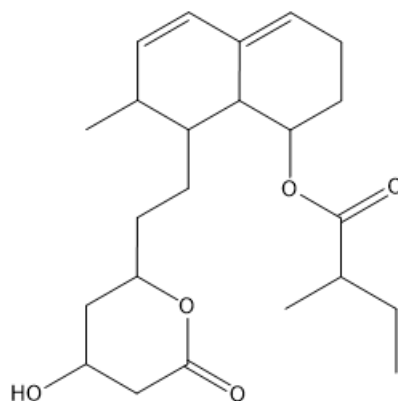
mevastatin
