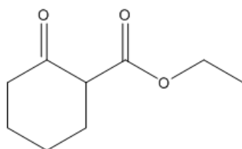
B - ketoester
