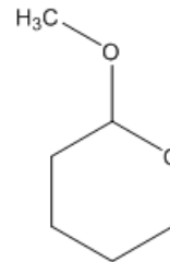
acetal
