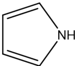
pyrrole
