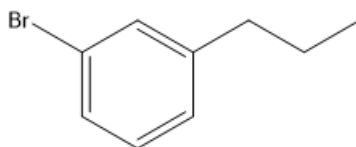
1-bromo-3-propylbenzene
