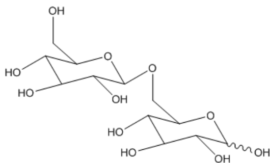
gentiobiose
